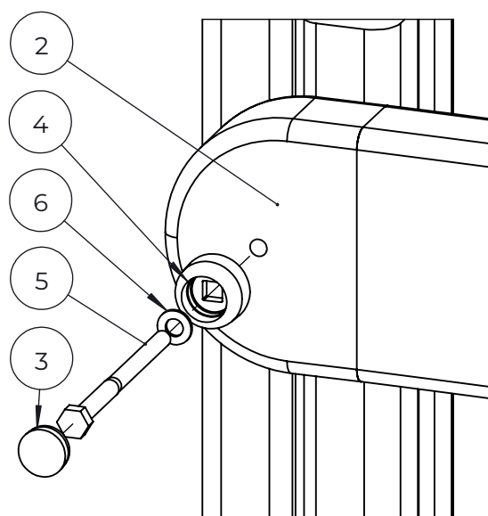
DET 4
