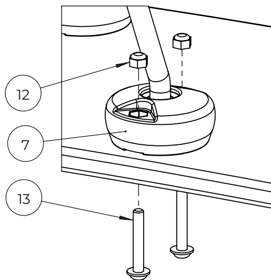
DET 4
