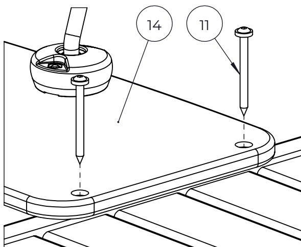
DET 3
